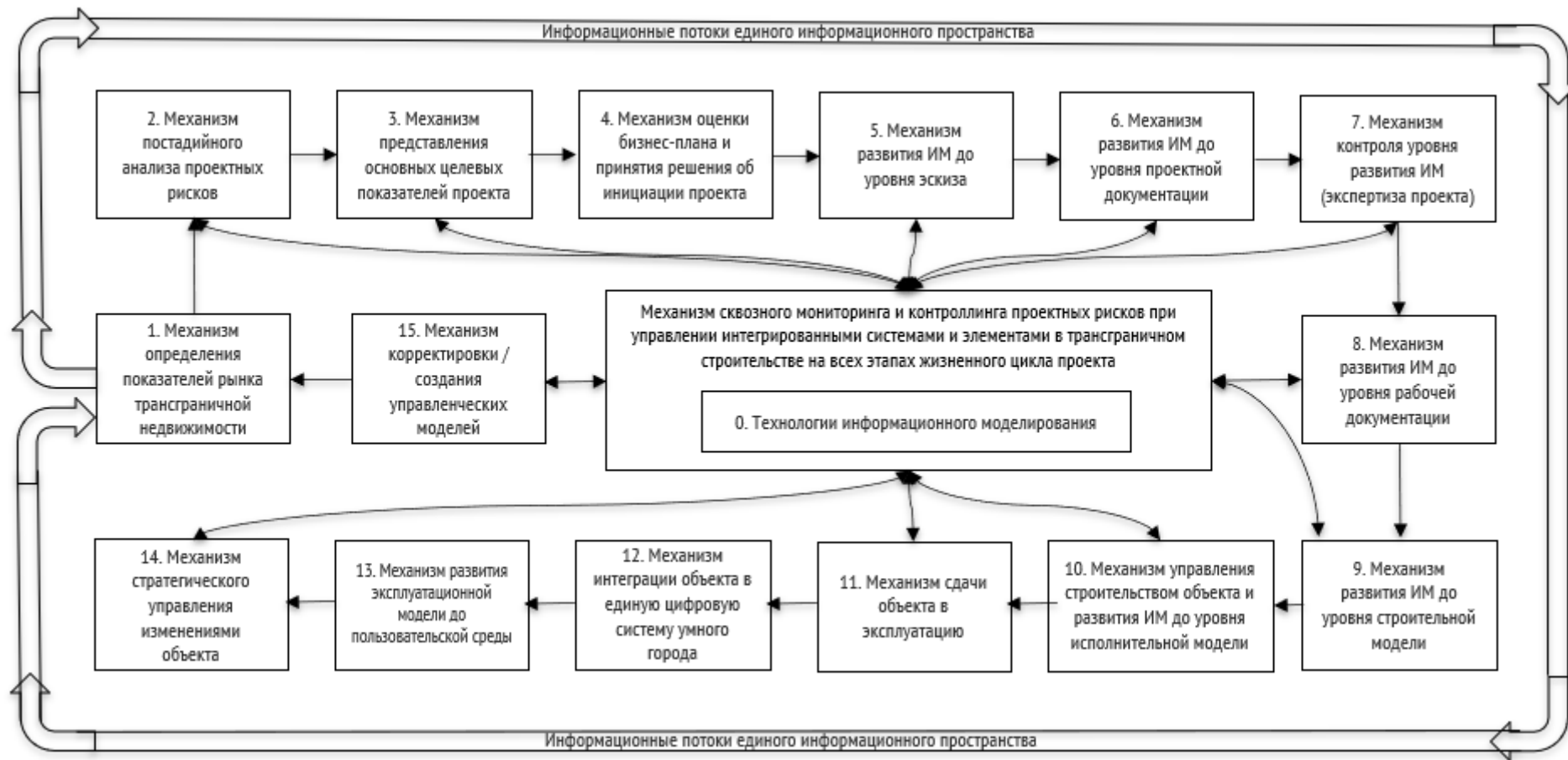
Рисунок 2. Модель управления трансграничным девелоперским проектом в разрезе проектных стадий жизненного цикла.
